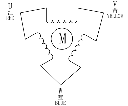
接线图/WIRING DIAGRAM
